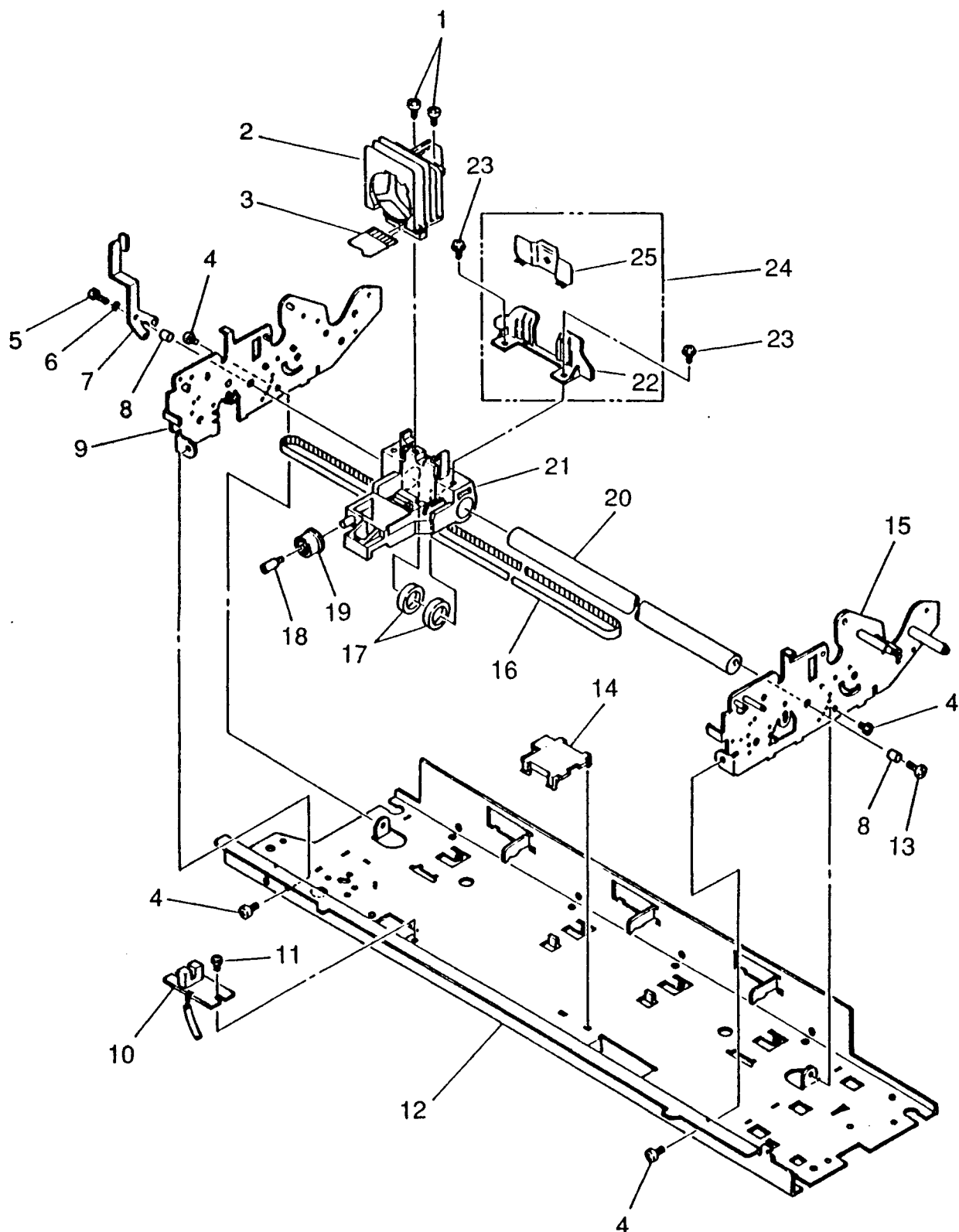
FIGURA 9-7 Accessori del Telaio III (922N) FIGURE 9-7 Chassis III (922N)
