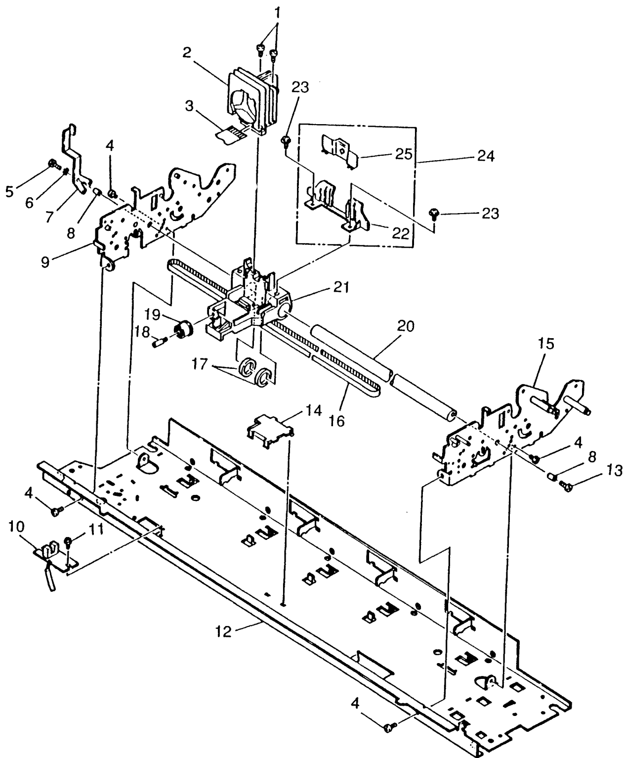
FIGURA 9-8 Accessori del Telaio III (923) FIGURE 9-8 Chassis III (923)
