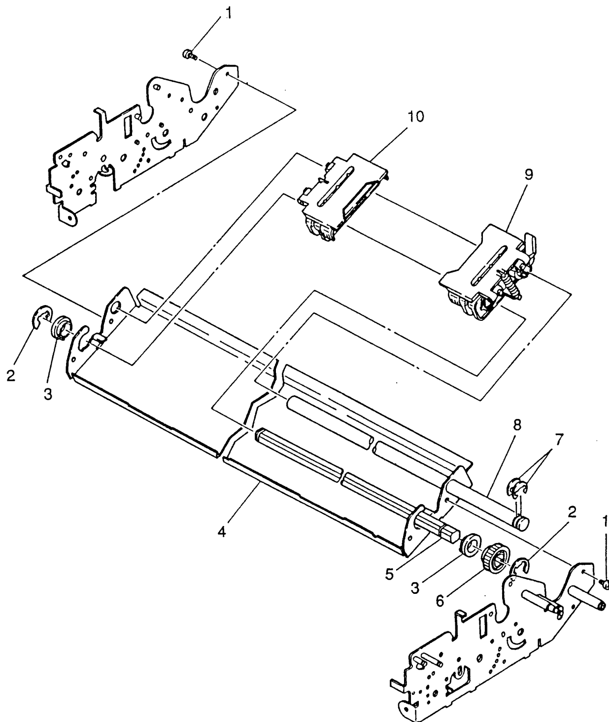
FIGURA 9-14 Sistema di Avanzamento a trattori (922N) FIGURE 9-14 Tractor Feed (922N)
