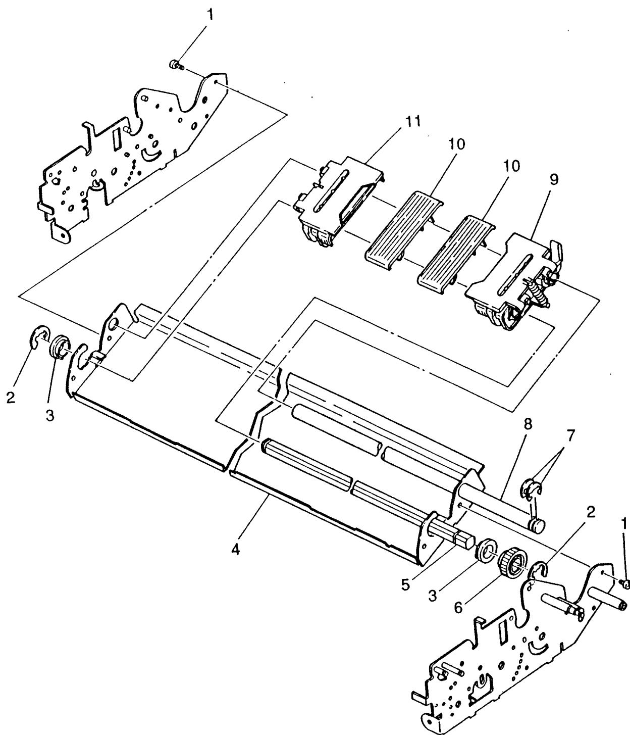
FIGURA 9-15 Sistema di Avanzamento a Trattori (923) FIGURE 9-15 Tractor Feed (923)
